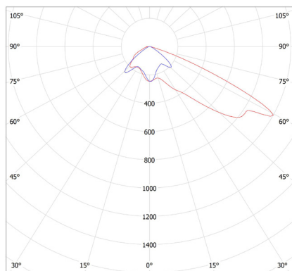
cd/klm — C0 - C180 — C90 - C270 Асимметрик (AS1)
